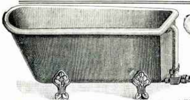
BAIGNOIRE fonte émaillée blanc, extérieur peinture blanche unie, avec soupape, coudé de trop-plein et siphon. Longueur totale 1 m 60, largeur 0 m 77 . . . . . 190. *
