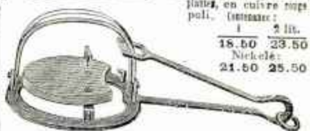
PIEGES en fer - palette bois. Long. totale: 0m38 0m35 0m38 0m43 0m44 Prix: . . . 3.10 2.95 4.95 6.25 11.25
