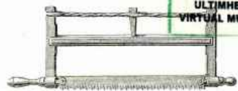
SCIE à refendre, monture cormier. Longueur de la lame 0 m 60 0 m 65 0 m 70 Prix 3.60 3.90 4.25
