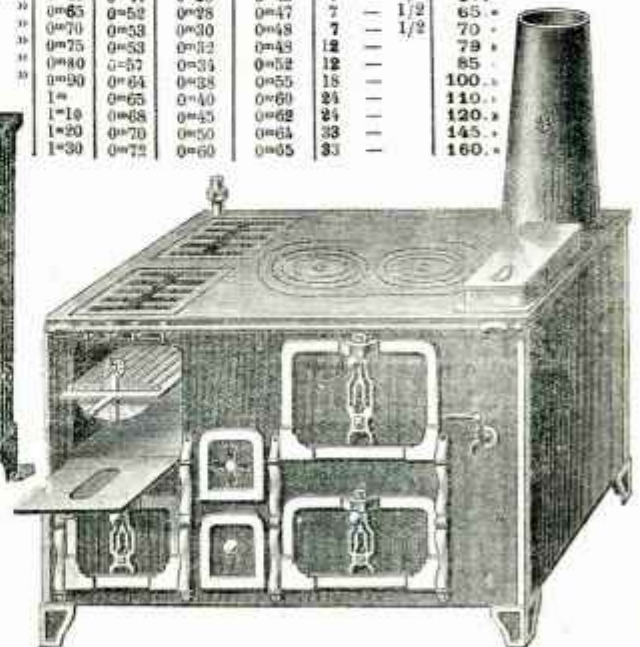
FOURNEAU tôle et fonte mixte, pour le charbon et le gaz, four à rôtir stove chaudière émaillée.
