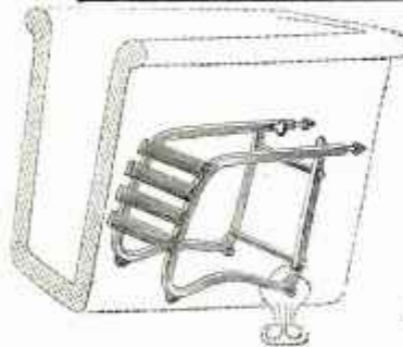
CALE-PIEDS , cuivre nickelé, traverses pitchpin verni.
