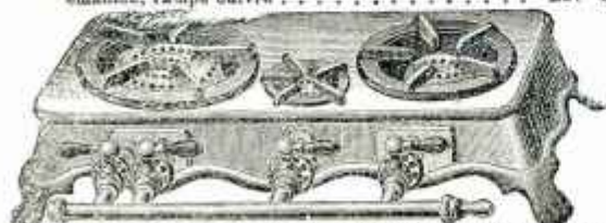
FOURNEAU A GAZ en fonte émaillée, à 3 feux et 2 robinets. Longueur totale 0 m 56, largeur 0 m 26, rampe cuivre. . . . . 19.50
