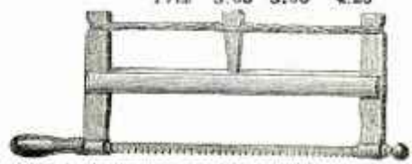
SCIE à chantourner, monture cormier. Longueurs 0 m 50 0 m 55 0 m 60 0 m 65 Prix 2.75 2.90 3.10 3.50
