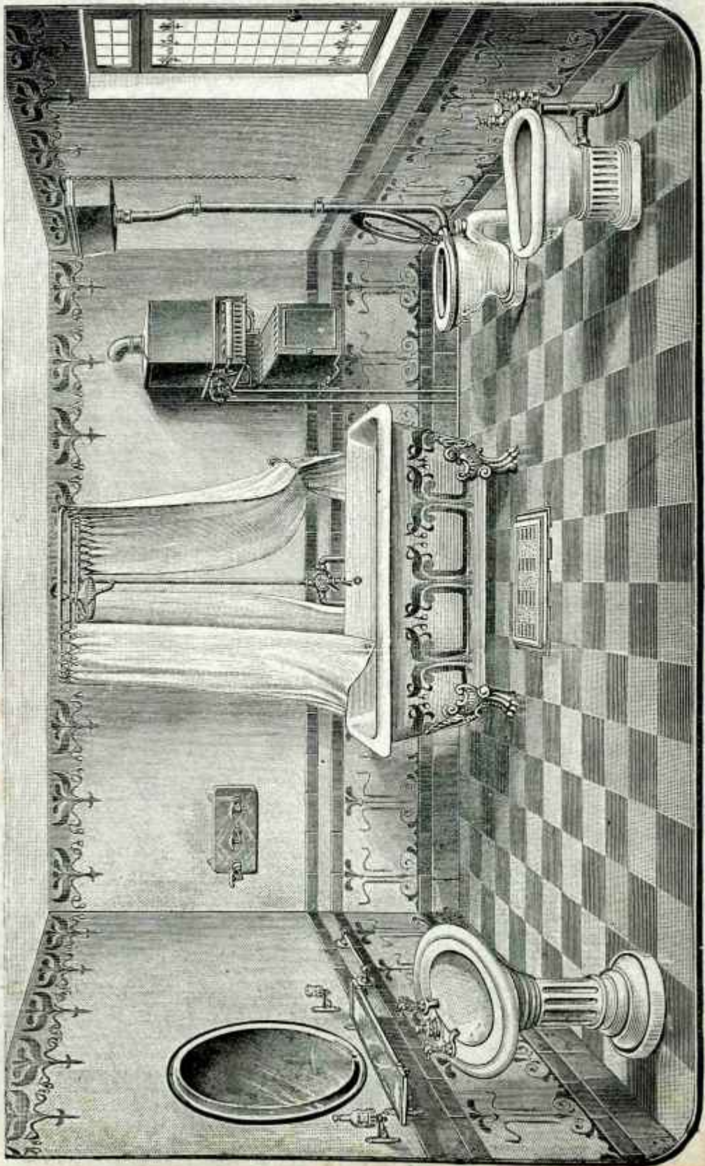
TYPE D'INSTALLATION D'UNE SALLE DE BAINS AU GAZ AVEC DOUCHE OU PLOIE, COMMANDE DU CHAUFFE-GAISE ET DE LA VIDANGE PAR LA MANŒUVRE DU ROBINET MITIGEUR
