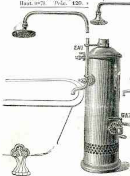
CHAUFFE-BAINS instantané à circulation, au gaz, avec colonne à douches, en cuivre jaune poli. Appareil en tôle galvanisée vernie. 195. * Le même, entièrement en cuivre. 235. * Le même en tôle, sur la colonne à douches, déversoir ordinaire. . . . . 140. *
