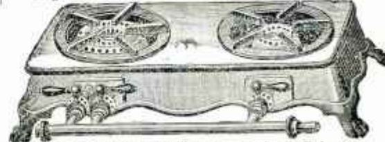
FOURNEAU A GAZ fonte émaillée, rampe cuivre poli, longueur totale 0 m 50, larg. 0 m 26, à 2 trous et 3 robinets. . . 16. » Le même, à 3 robinets. . . . . Preis 19.50
