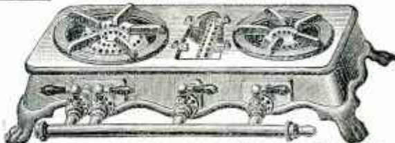
FOURNEAU A GAZ en fonte émaillée, rampe cuivre, 2 feux pour cuisine et 1 pour fer à repasser. Long. totale 0 m 55. larg. 0 m 26 . . . . . 20.50
